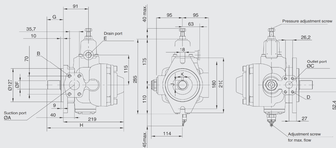
PVV101-2-31 / -40 / -50 (FS / US)
