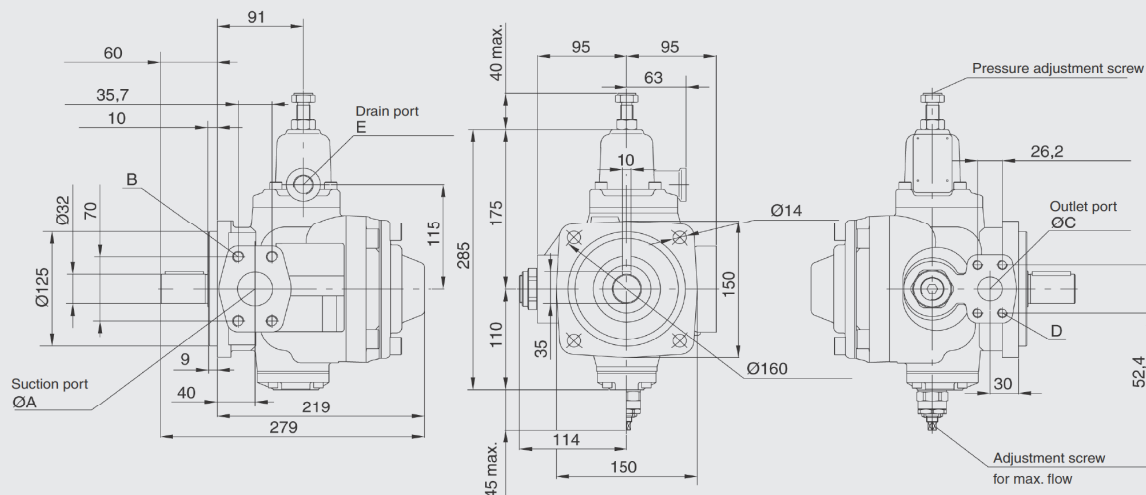
PVV101-2-31 / -40 / -50 (F / F UNC)
